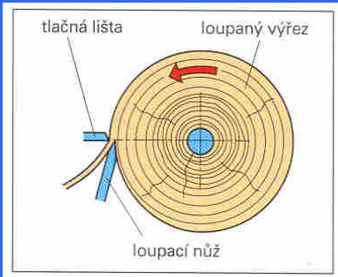
Loupání dýhy (centrické)
